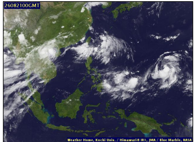
ภาพถ่ายดาวเทียม วันที่ ๒๑ ส.ค. ๒๕๖๙ เวลา ๐๗.๐๐ น.
